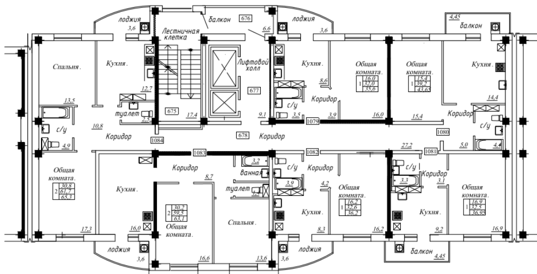
Схема блокировки
